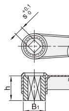
方孔固定
