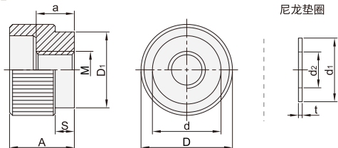
尼龙垫圈
