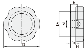
内螺纹 SJD02
