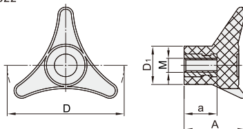
防静电 SJB22
