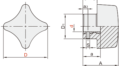
销钉固定型 SJA51
