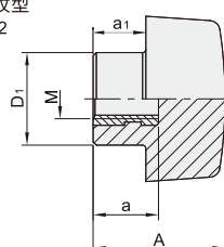
内螺纹型 SJA53
