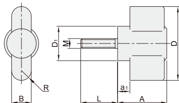
外螺纹型 SJA41
