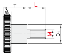
带台阶外螺纹型
