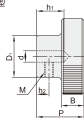
螺钉锁紧型 SGE31 SGE32 SGE33
