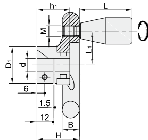
夹紧位置详细尺寸
