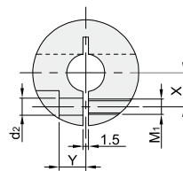
夹紧位置详细尺寸
