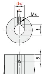
键槽孔型
