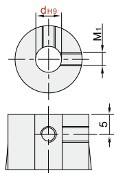
■ 内孔 d 形状选择 螺钉锁紧型
