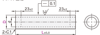
OCF06 立柱
