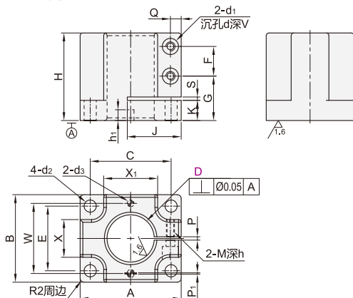
OCF01 底座
