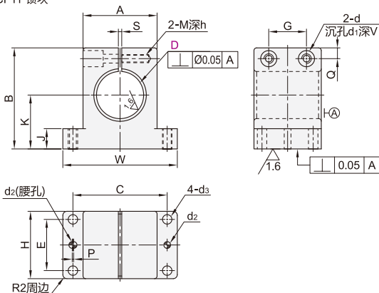
OCF11 锁块
