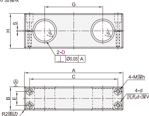
OCF16 加强块
