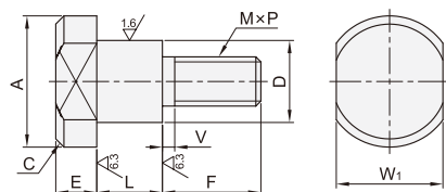
头部切割型 MYD21/23/24/25/22/26
