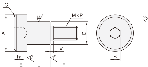
内六角孔型 MYD11/13/14/15/12/16
