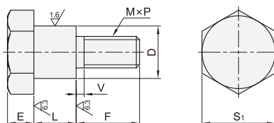
六角头型 MYD31/32/36/41/42/46
