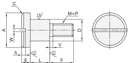
头部切割型 MYD21/23/24/25/22/26
