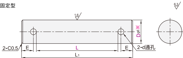
■ 开口销固定型
