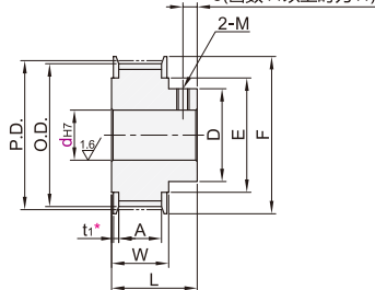
带轮形状: B形
