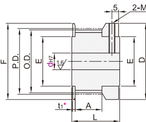
带轮形状:K型
