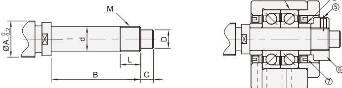
参考轴端加工尺寸
