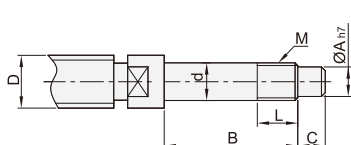
参考轴端加工尺寸
