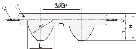
FCX01/05 标准型 皮带类型:S5M/S8M
