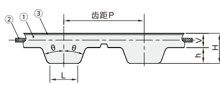
FCX04/08 两面贴布型
