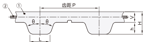
FCX01/05 标准型 皮带类型:S5M/S8M
