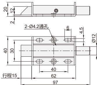
腰孔型 FAY32
