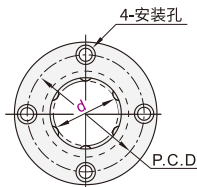
圆法兰型
