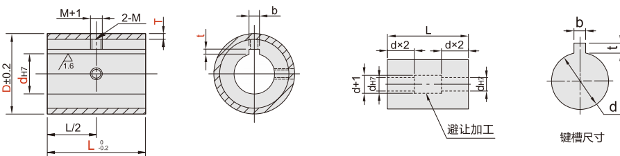
带螺纹孔式
