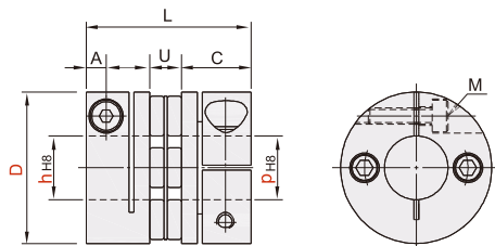
CDE01 单膜片
