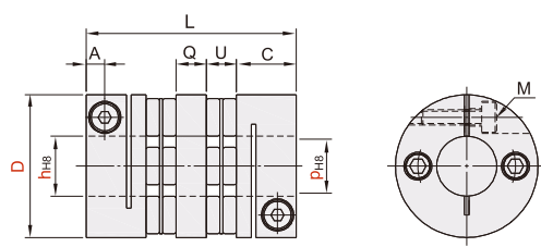
CDE21 双膜片
