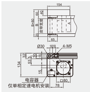
■ 调速\定速\变频电机尺寸(参考值)
