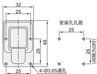
无锁型·方型 HBA31
