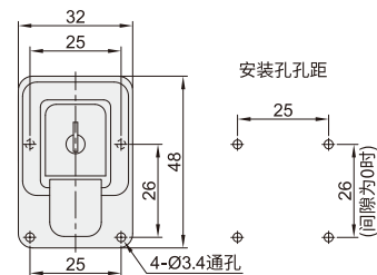
带锁型·方型 HBA33
