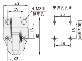
无锁型·碟型 HBA32
