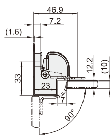
安装尺寸图
