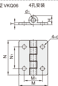
圆孔型 VKQ06
