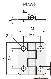
圆孔+腰孔型 VKK03
