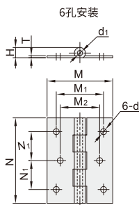
圆孔错位型 VKK02
