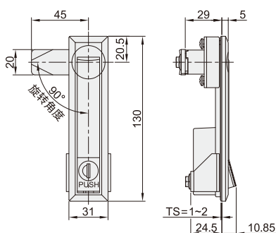
XAD29锁舌形状
