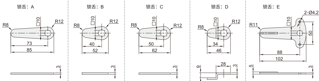
XAD29锁舌形状
