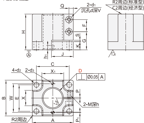
AZD02 底座
