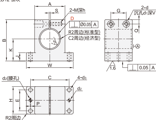
AZD12 锁块
