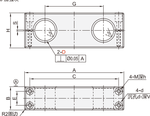
AZD16 加强块
