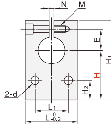
开口型 ZFS01/02/06/08
