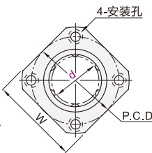
法兰型
