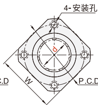
方法兰型 ELW21MX ELW22MX
