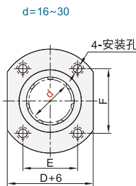
对边法兰型 ELW31MX ELW32MX
