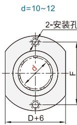
对边法兰型 ELW31MX ELW32MX
