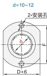
对边法兰型 ELU31MX ELU32MX
