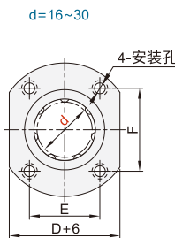
对边法兰型 ELU31MX ELU32MX
