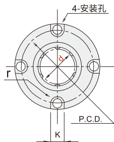
圆法兰型
