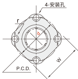
方法兰型
