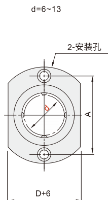
两面切割/法兰型
