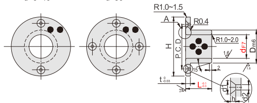
FDK02 锥孔型
