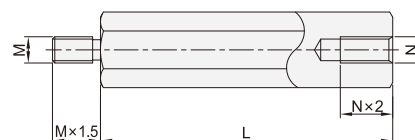
L尺寸螺纹指定型 OBE11/12/13/16
