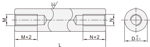
螺纹指定型 OAA21/22/23/26/28
