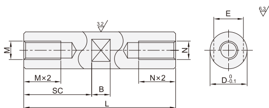
螺纹指定带扳手槽型 OAA31/32/33/36/38
