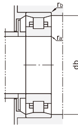
(安装图)
