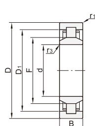
内圈无挡边 BDN01
