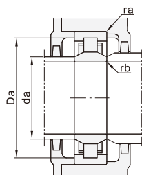
(安装图)
