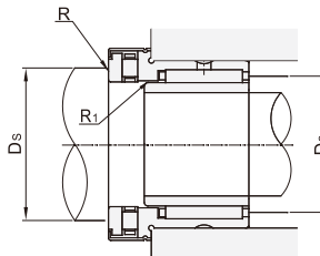
(安装图)
