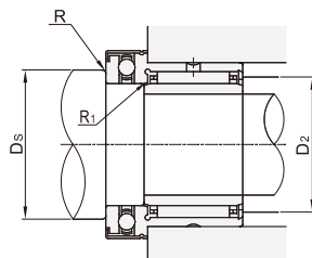
(安装图)
