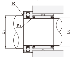
(安装图)
