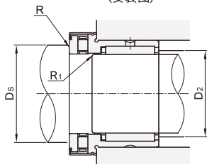
(安装图)
