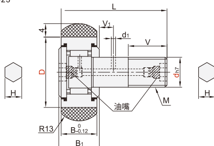
头部螺纹部内六角孔(d12~16) BCC22 BCC23
