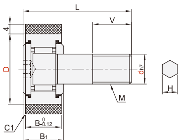
圆柱型 头部内六角孔(d5~10) BCC41 BCC43
