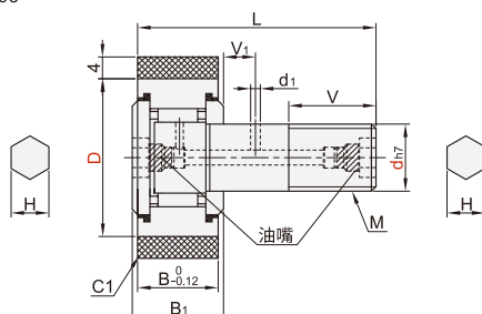
头部螺纹部内六角孔(d12~16) BCC02 BCC03
