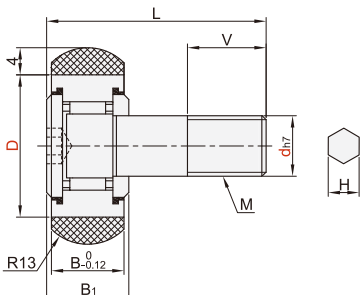
球面型 头部内六角孔(d5~10) BCC61 BCC63
