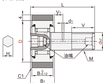
头部螺纹部内六角孔(d12~16) (带密封圈)
