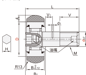
头部螺纹部内六角孔(d12~16) (带密封圈)
