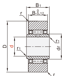
圆柱型BCN01/02
