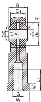
内螺纹 BGJ01/02
