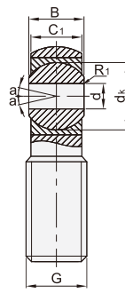
外螺纹 BGJ11/12
