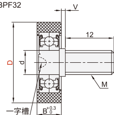
长螺纹型
