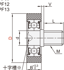
外螺纹型
