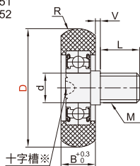
外螺纹型
