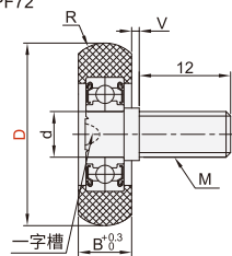
长螺纹型
