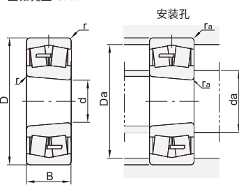
圆锥孔型 CAK
