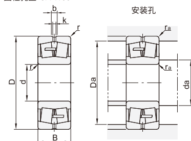
圆柱孔型 CA-W33
