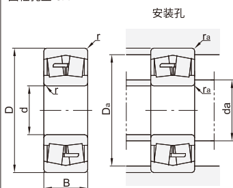
GBSR01 圆柱孔型 CA
