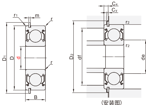
(安装图)
