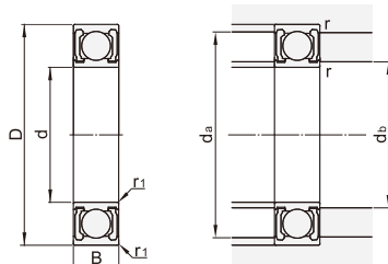
非接触式橡胶密封圈型
