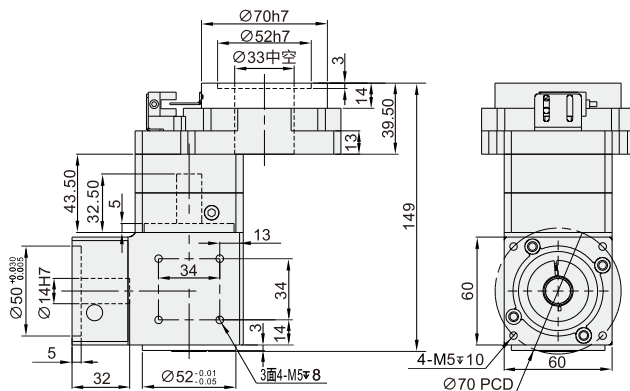
K向视图
