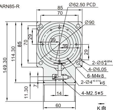
ARN85-R
