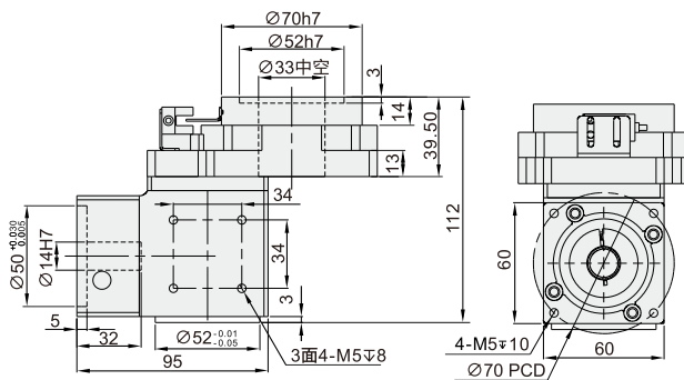
K向视图
