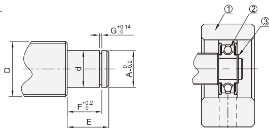
参考轴端加工尺寸
