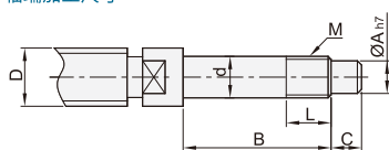
参考轴端加工尺寸
