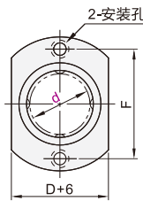
对边法兰型
