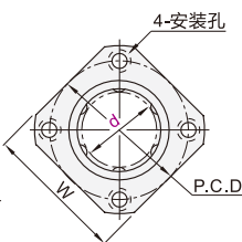
方法兰型
